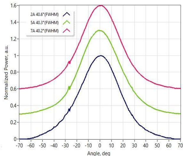
快轴远场
