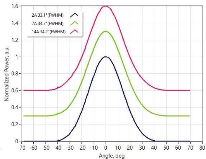
快轴远场
